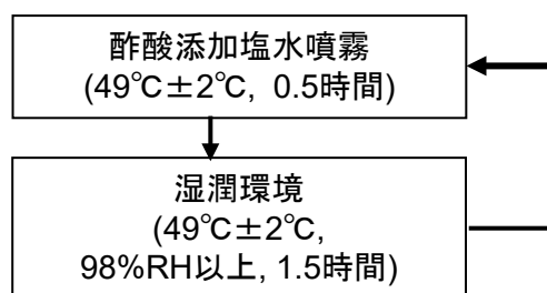
図2 SWAAT 試験の温湿度サイクル
