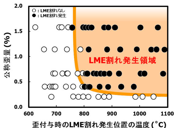
図2 LM-CAST試験™による980GA鋼板のLME割れ感受性評価例（LSTR）
