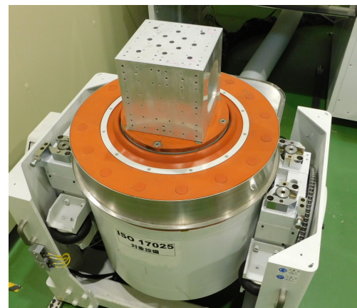
図 動電型振動試験機(加振力40 kN)
