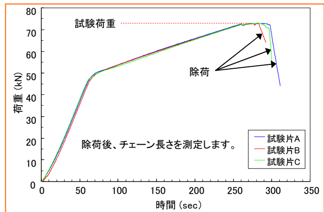
荷重-時間線図
